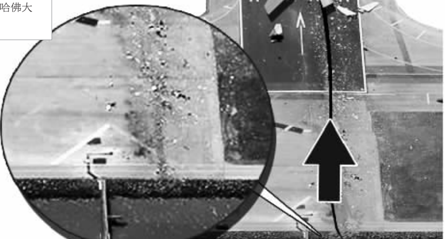
1 降落时撞上防海墙,飞机断裂
